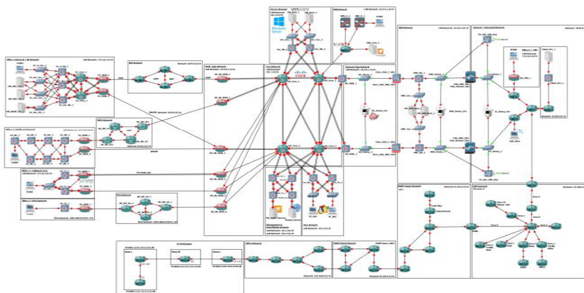
Рис.7. Интерфейс GNS3 – лабораторная работа
